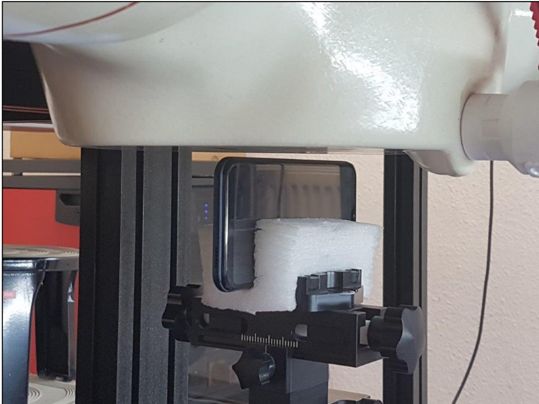
Photo 11: Position d'essai face du côté gauche contre le corps (distance 5 mm)
