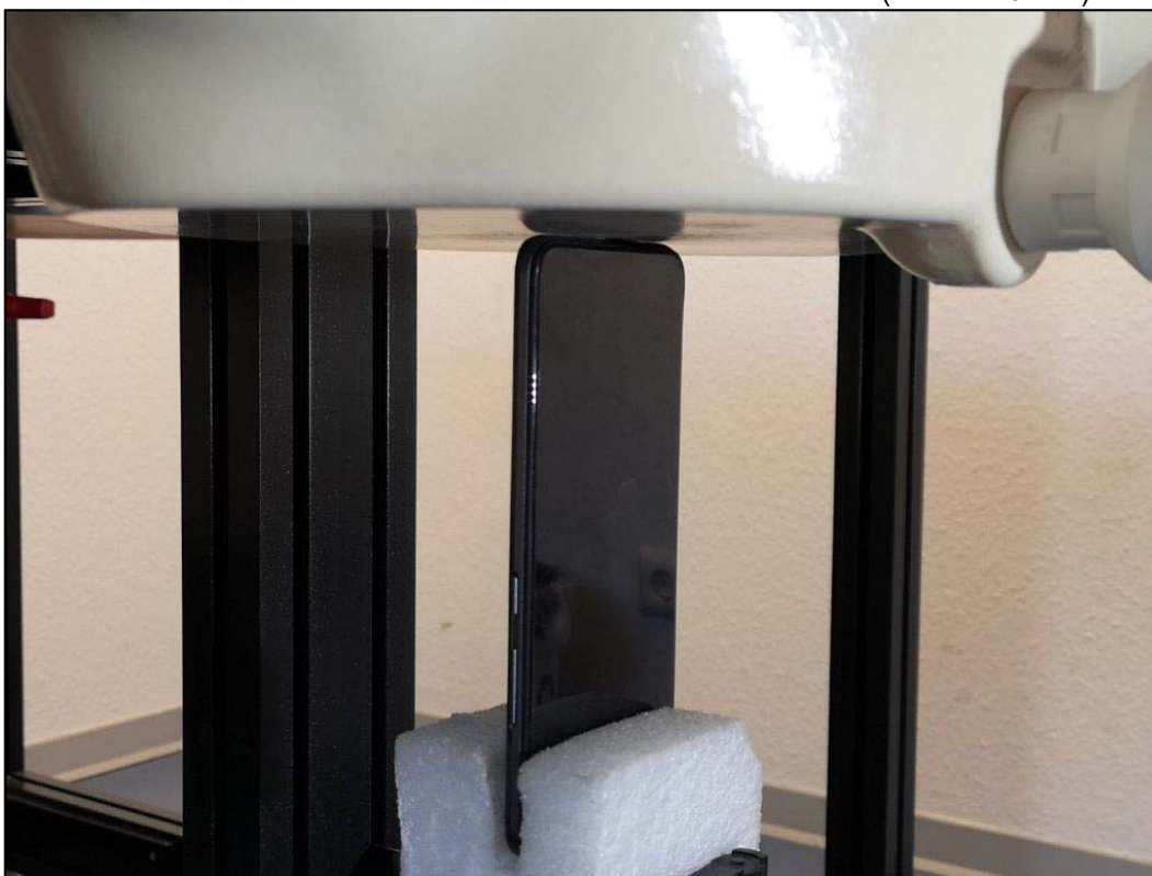
Photo 11: Position d'essai face du dessous contre le membre (distance 0 mm)
