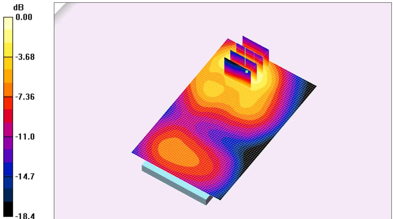
Fig. 9 : Distribution du DAS en GSM-GPRS 1800: canal 512 (1710.2 MHz) face arrière à 1.5cm du fantôme
