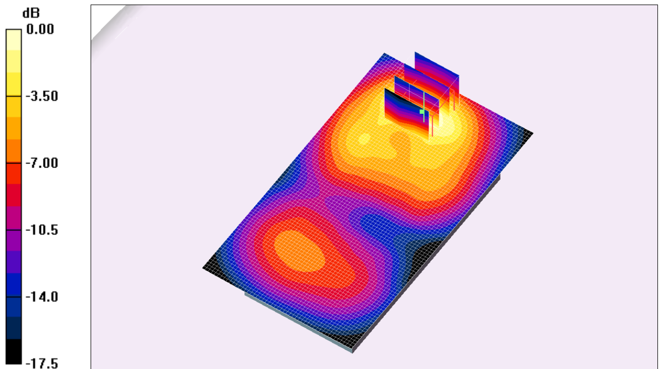
Fig. 13 : Distribution du DAS en LTE 1800: canal 19300 (1720.0 MHz) face arrière à 1.5cm du fantôme
