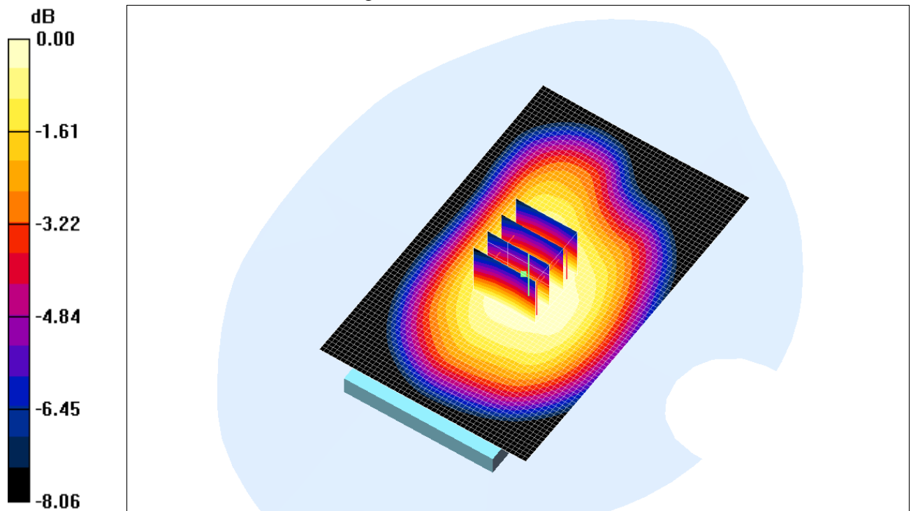
Fig. 8 : Distribution du DAS en GSM-GPRS 900: canal 975 (880.2 MHz) face arrière à 1.5cm du fantôme
