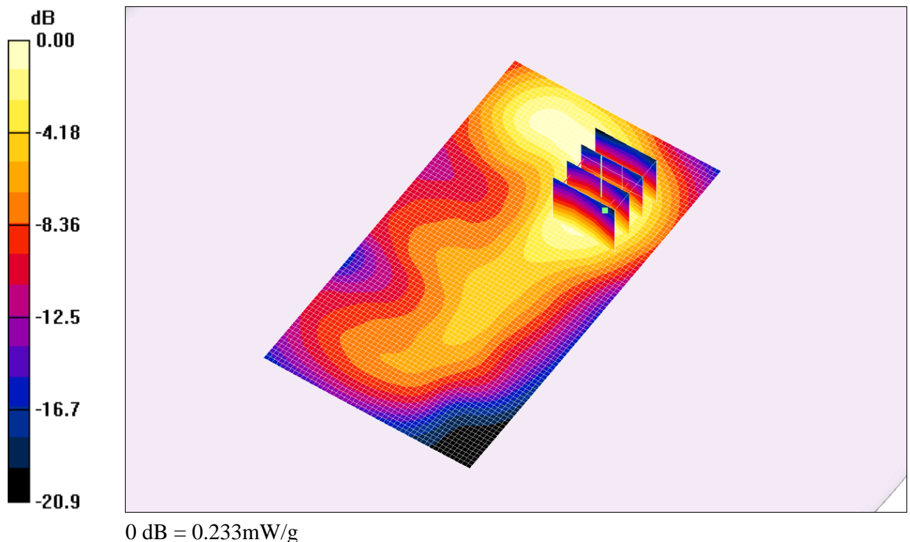
Fig. 14 : Distribution du DAS en LTE 2600: canal 21425 (2567.5 MHz) face avant à 1.5cm du fantôme
