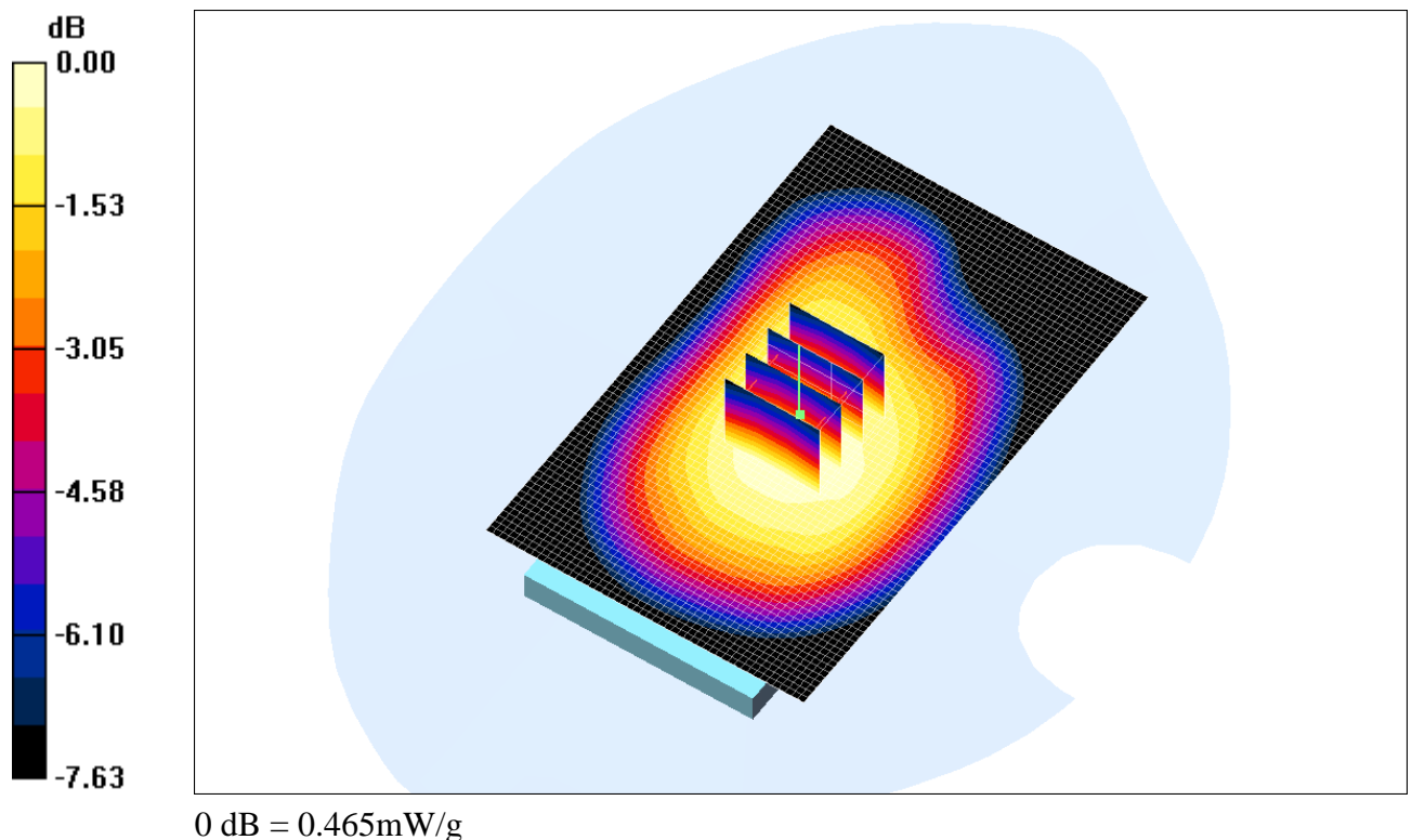
Fig. 10 : Distribution du DAS en WCDMA 900: canal 2863 (912.6 MHz) face arrière à 1.5cm du fantôme
