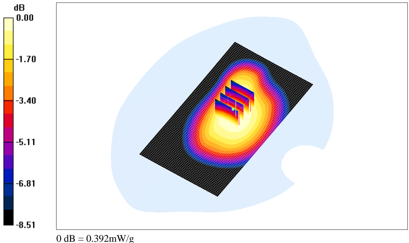
Fig. 12 : Distribution du DAS en LTE 800: canal 24300 (847.0 MHz) face arrière à 1.5cm du fantôme
