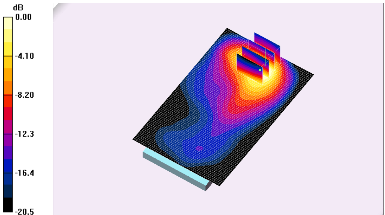
Fig. 9 : Distribution du DAS en GSM-GPRS 1800: canal 885 (1784.8 MHz) face avant à 0.5cm du fantôme
