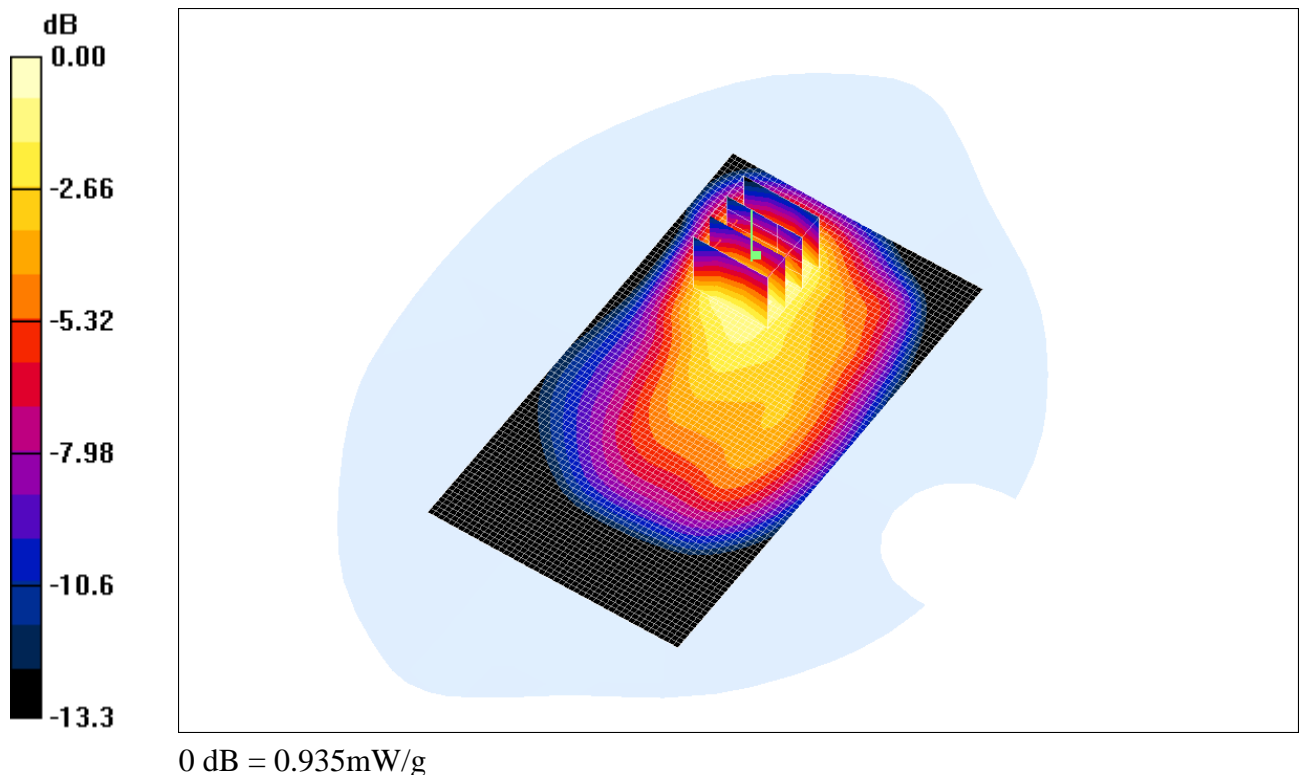
Fig. 12 : Distribution du DAS en LTE 800: canal 24300 (847.0 MHz) face arrière à 0.5cm du fantôme
