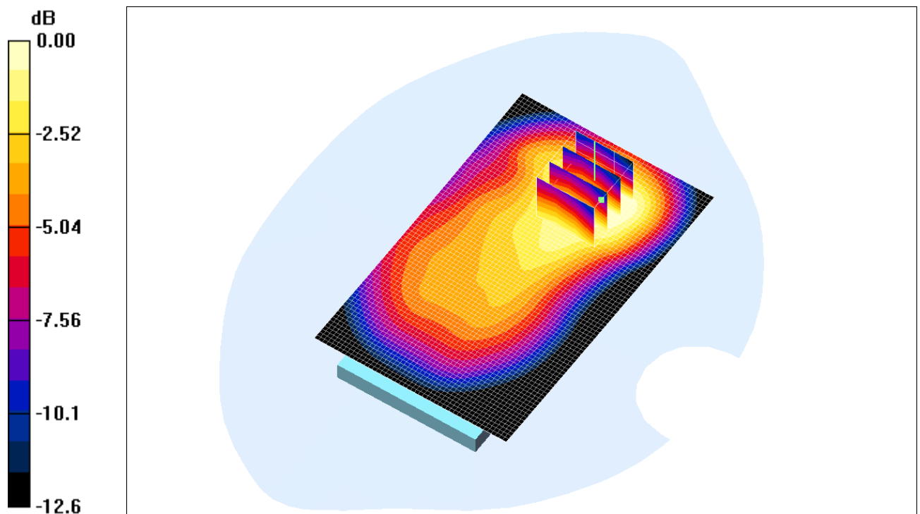
Fig. 10 : Distribution du DAS en WCDMA 900: canal 2712 (882.4 MHz) face avant à 0.5cm du fantôme
