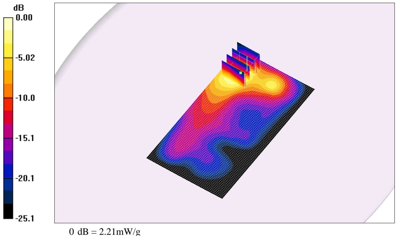
Fig. 14 : Distribution du DAS en LTE 2600: canal 21425 (2567.5 MHz) face arrière à 0.5cm du fantôme
