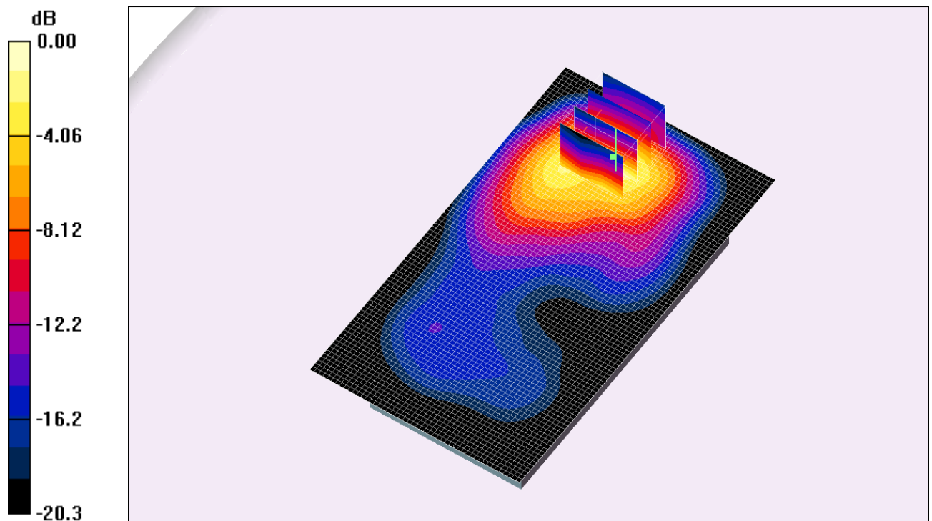
Fig. 13 : Distribution du DAS en LTE 1800: canal 19300 (1720.0 MHz) face arrière à 0.5cm du fantôme
