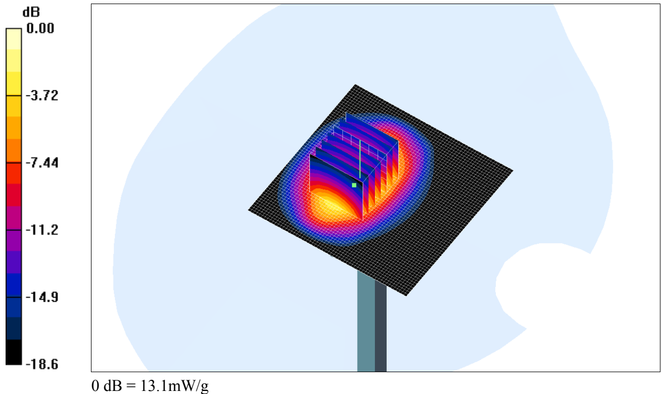
Fig. 5: Résultat de la vérification à 1950MHz
