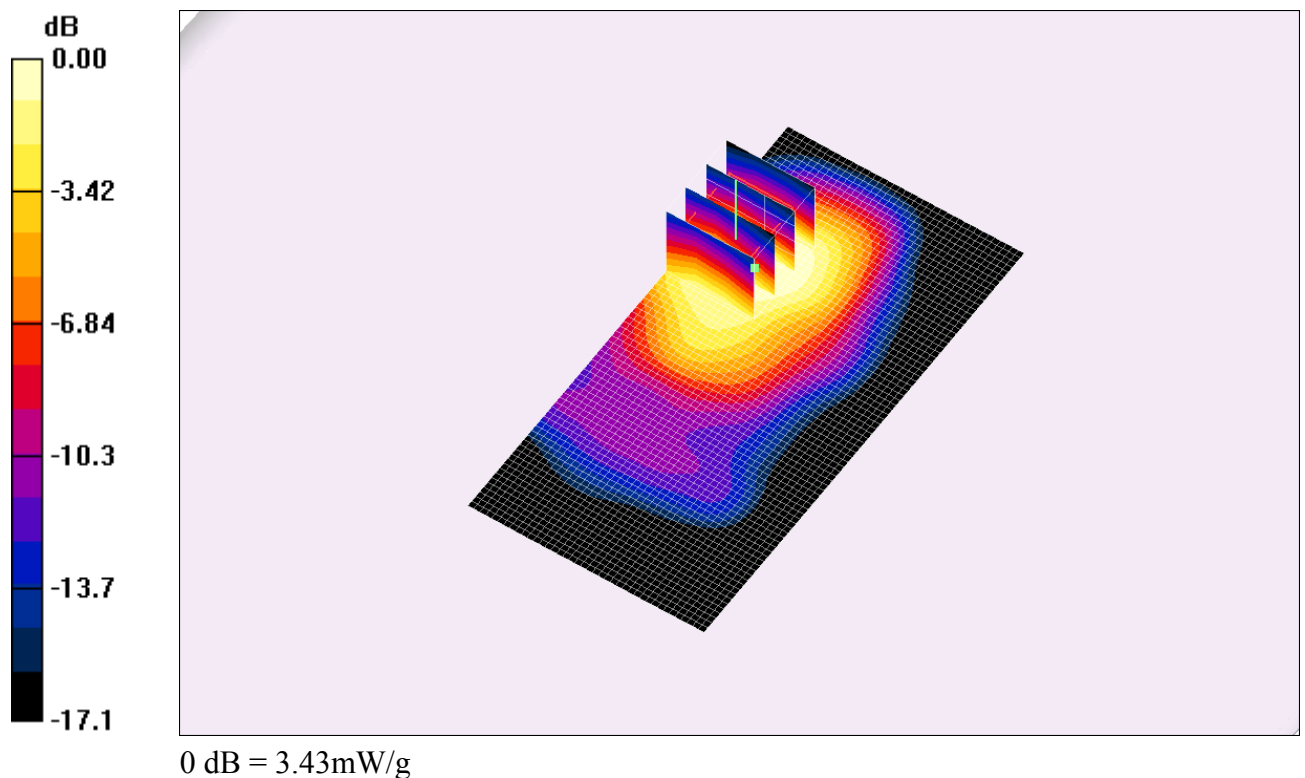
Fig. 7: Distribution du DAS en GSM-GPRS 1800: canal 885 (1784.8 MHz) face arrière à 0cm du fantôme
