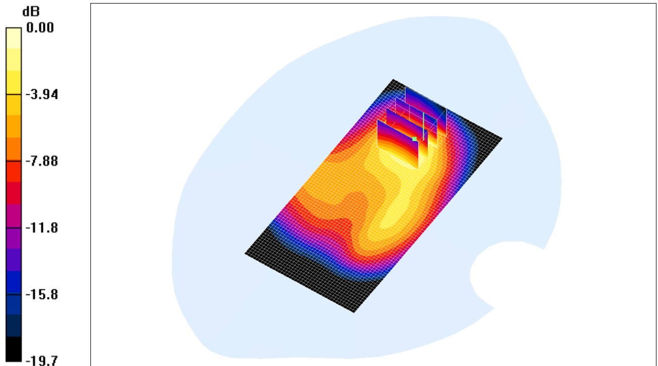
Fig. 6: Distribution du DAS en GSM-GPRS 900: canal 124 (914.8 MHz) face arrière à 0cm du fantôme
