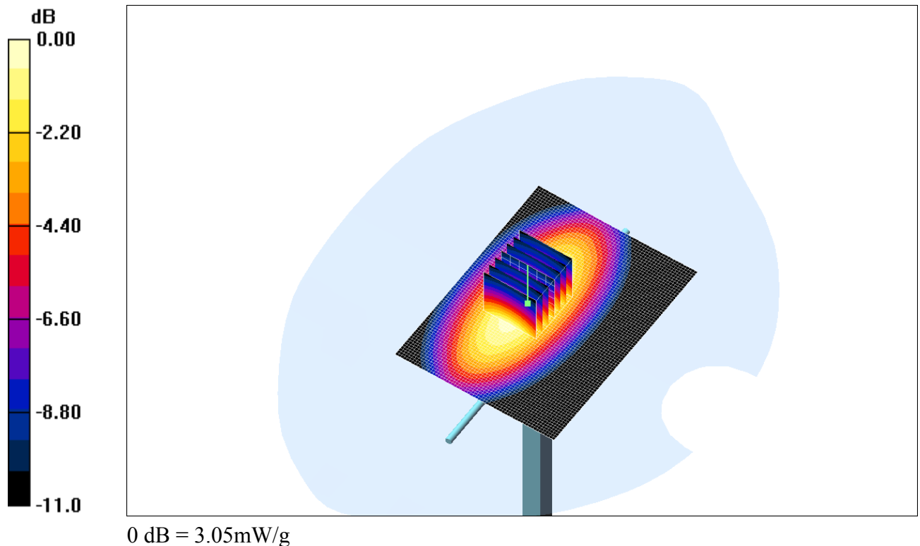
Fig. 3: Résultat de la vérification à 900MHz
