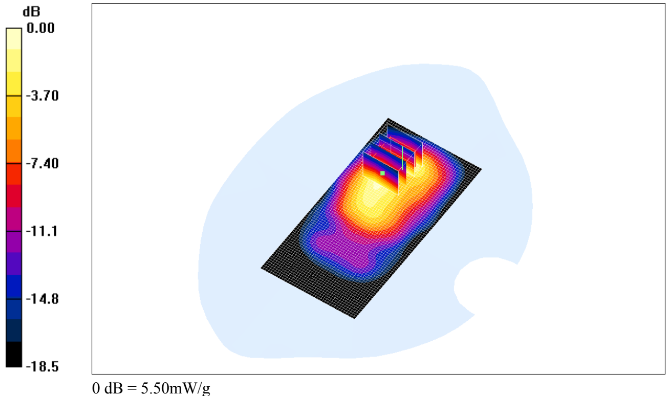
Fig. 9: Distribution du DAS en WCDMA 2100: canal 9888 (1977.6 MHz) face arrière à 0cm du fantôme
