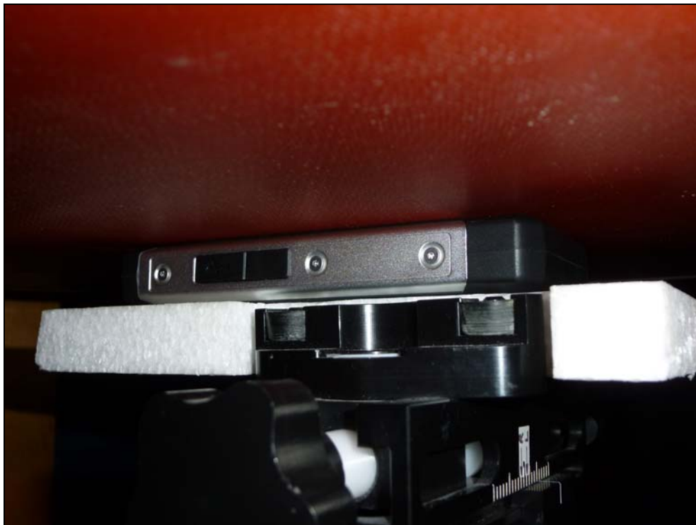
Fig. 12: Face avant à 0cm du fantôme ELI4
