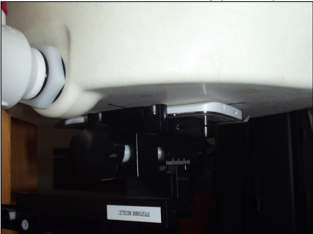
Photo 12: Position d'essai face avant contre le corps (distance 0 mm)
