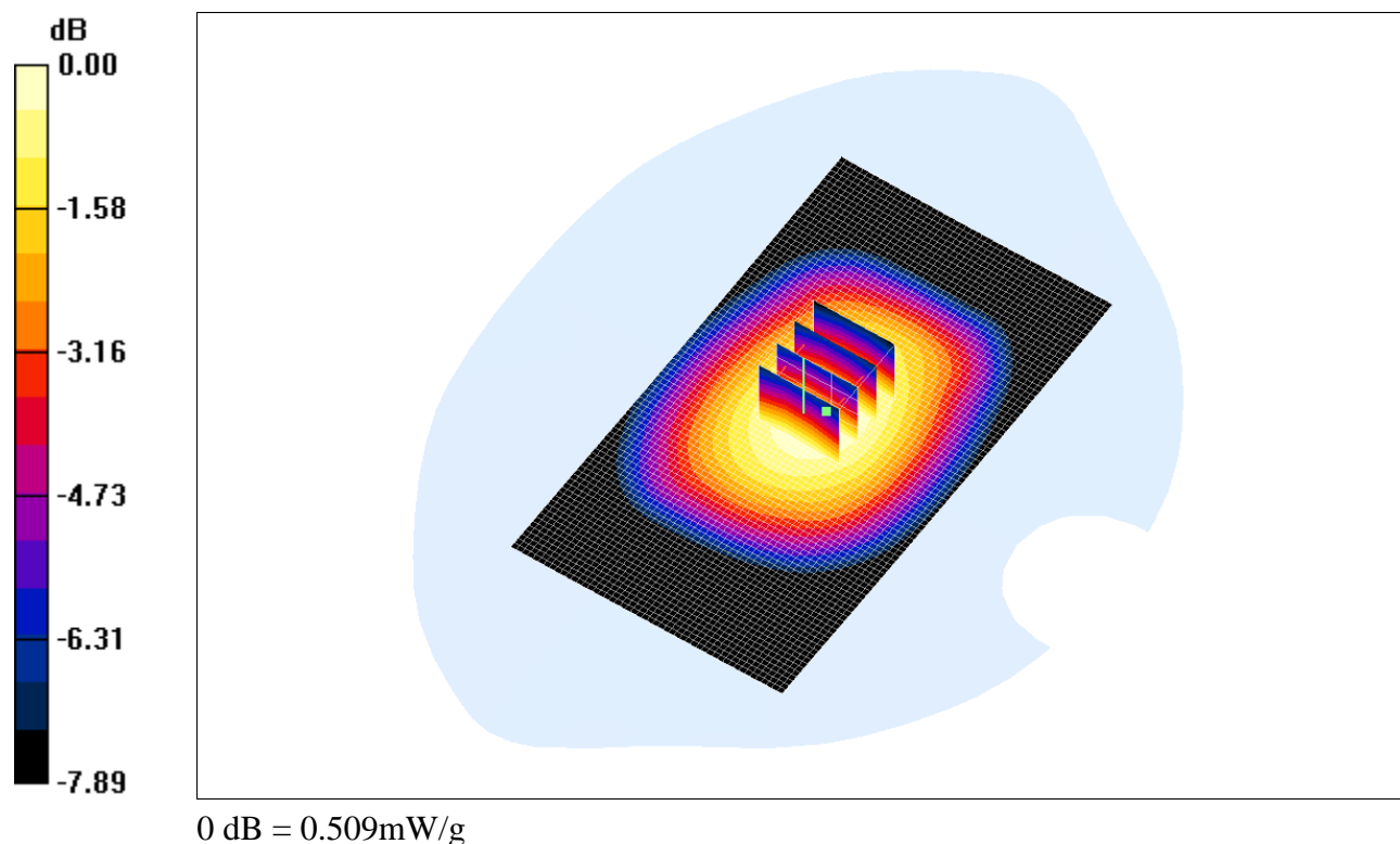
Fig. 12: Distribution du DAS en LTE 800: canal 24250 (842.0 MHz) face arrière à 1.5cm du fantôme
