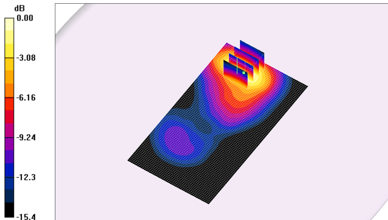
Fig. 9: Distribution du DAS en GSM-GPRS 1800: canal 885 (1784.8 MHz) face arrière à 1.5cm du fantôme
