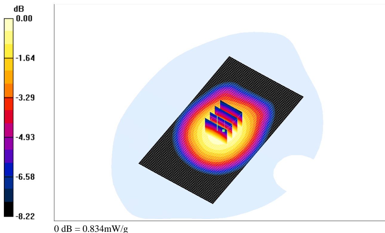
Fig. 8: Distribution du DAS en GSM-GPRS 900: canal 124 (914.8 MHz) face arrière à 1.5cm du fantôme
