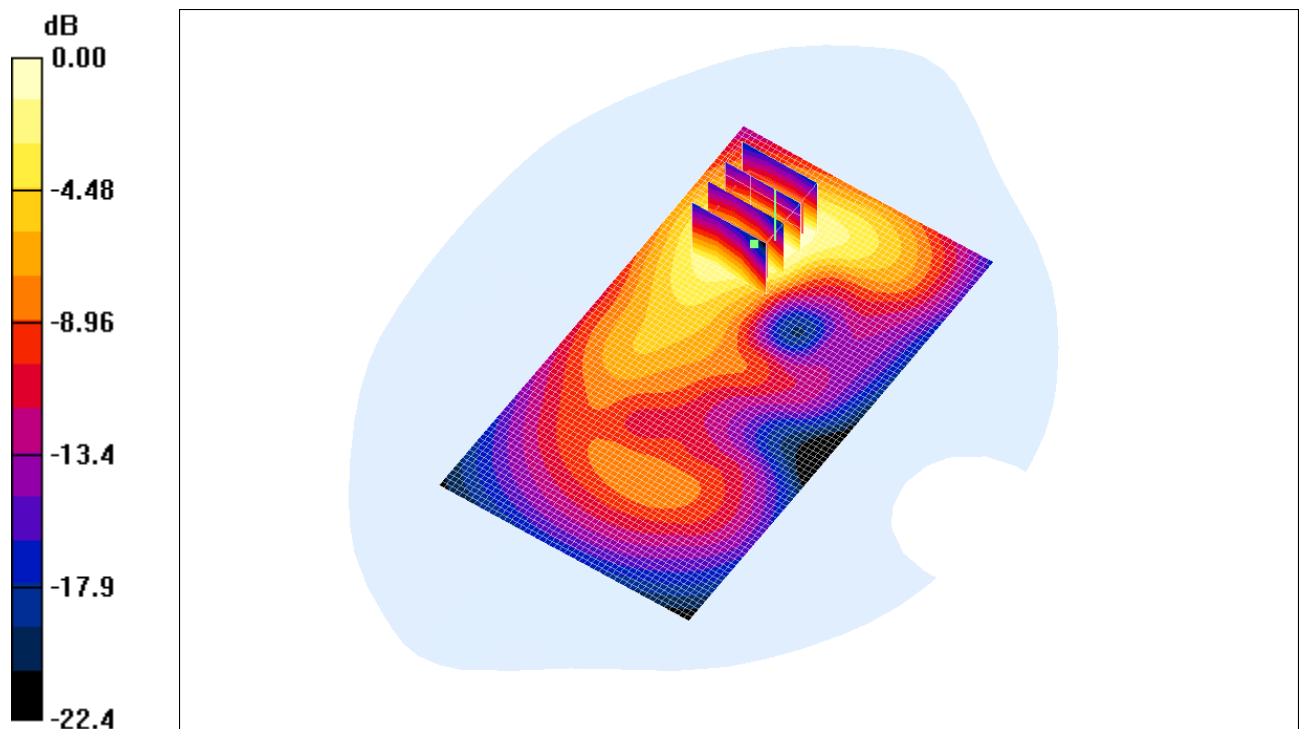
Fig. 14: Distribution du DAS en LTE 2600: canal 21100 (2535.0 MHz) face avant à 1.5cm du fantôme
