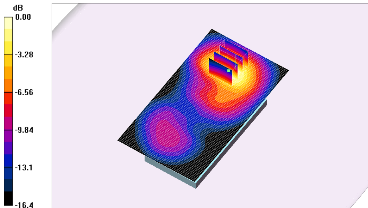
Fig. 13: Distribution du DAS en LTE 1800: canal 19575 (1747.5 MHz) face arrière à 1.5cm du fantôme
