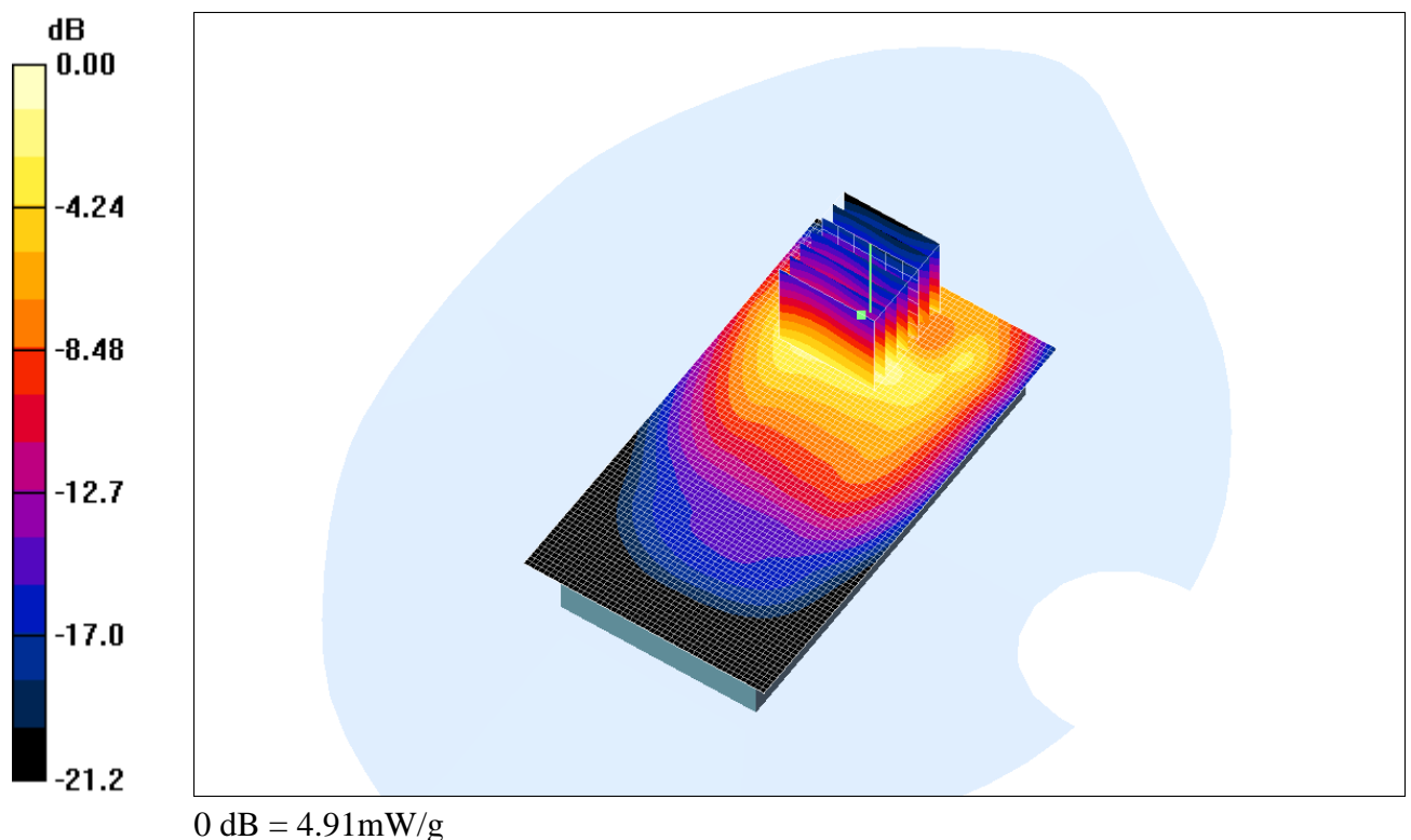
Fig. 7: Distribution du DAS en GSM-GPRS 1800: canal 699 (1747.6 MHz) face arrière à 0cm du fantôme
