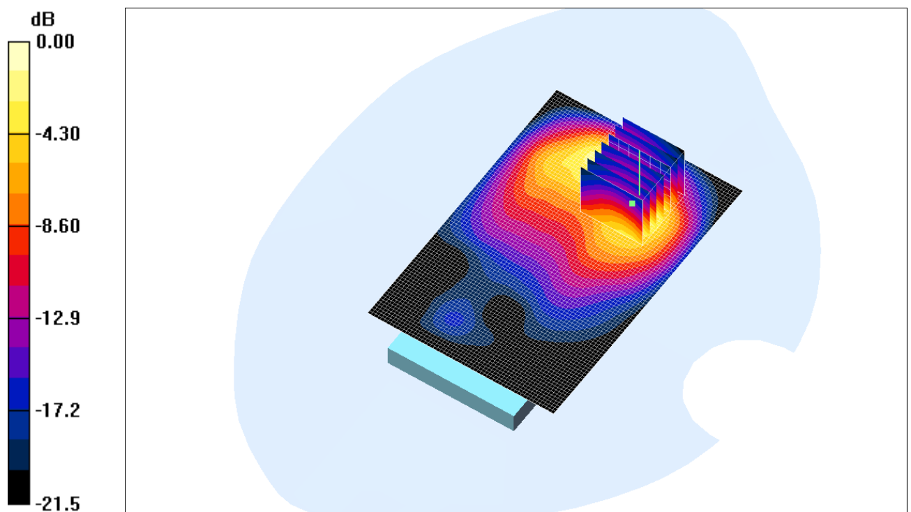
Fig. 9: Distribution du DAS en WCDMA 2100: canal 9750 (1950.0 MHz) face avant à 0cm du fantôme
