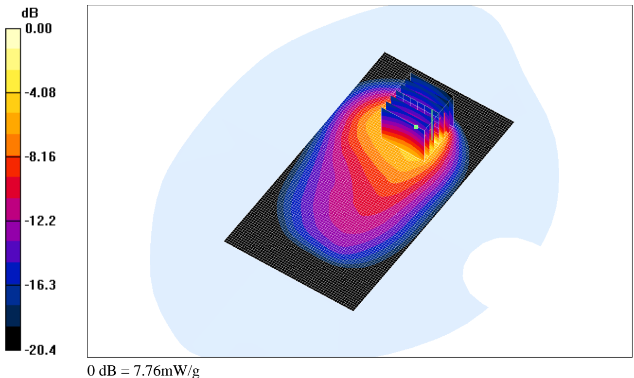
Fig. 8: Distribution du DAS en WCDMA 900: canal 2788 (897.6 MHz) face arrière à 0cm du fantôme
