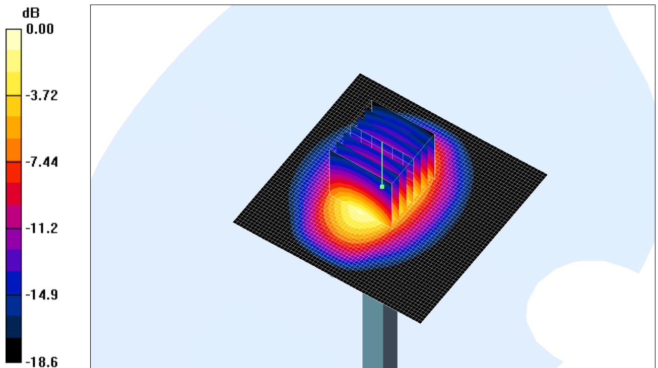
Fig. 5: Résultat de la vérification à 1950MHz
