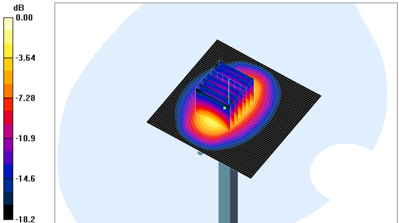
Fig. 4: Résultat de la vérification à 1800MHz
