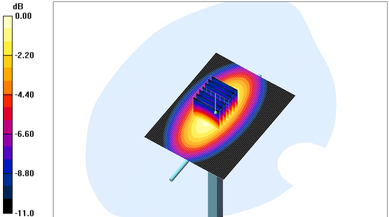
Fig. 3: Résultat de la vérification à 900MHz
