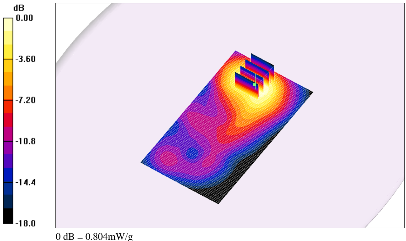
Fig. 14 : Distribution du DAS en LTE 2600: canal 20850 (2510.0 MHz) face avant à 1.5cm du fantôme
