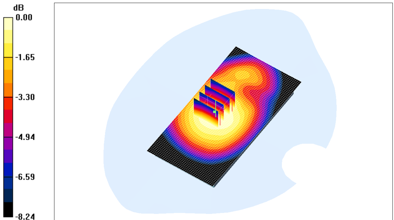
Fig. 10 : Distribution du DAS en WCDMA 900: canal 2788 (897.6 MHz) face arrière à 1.5cm du fantôme
