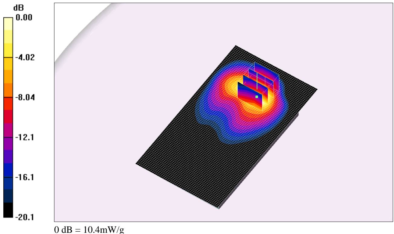
Fig. 13: Distribution du DAS en LTE 1800: canal 19225 (1712.5 MHz) face arrière à 0cm du fantôme
