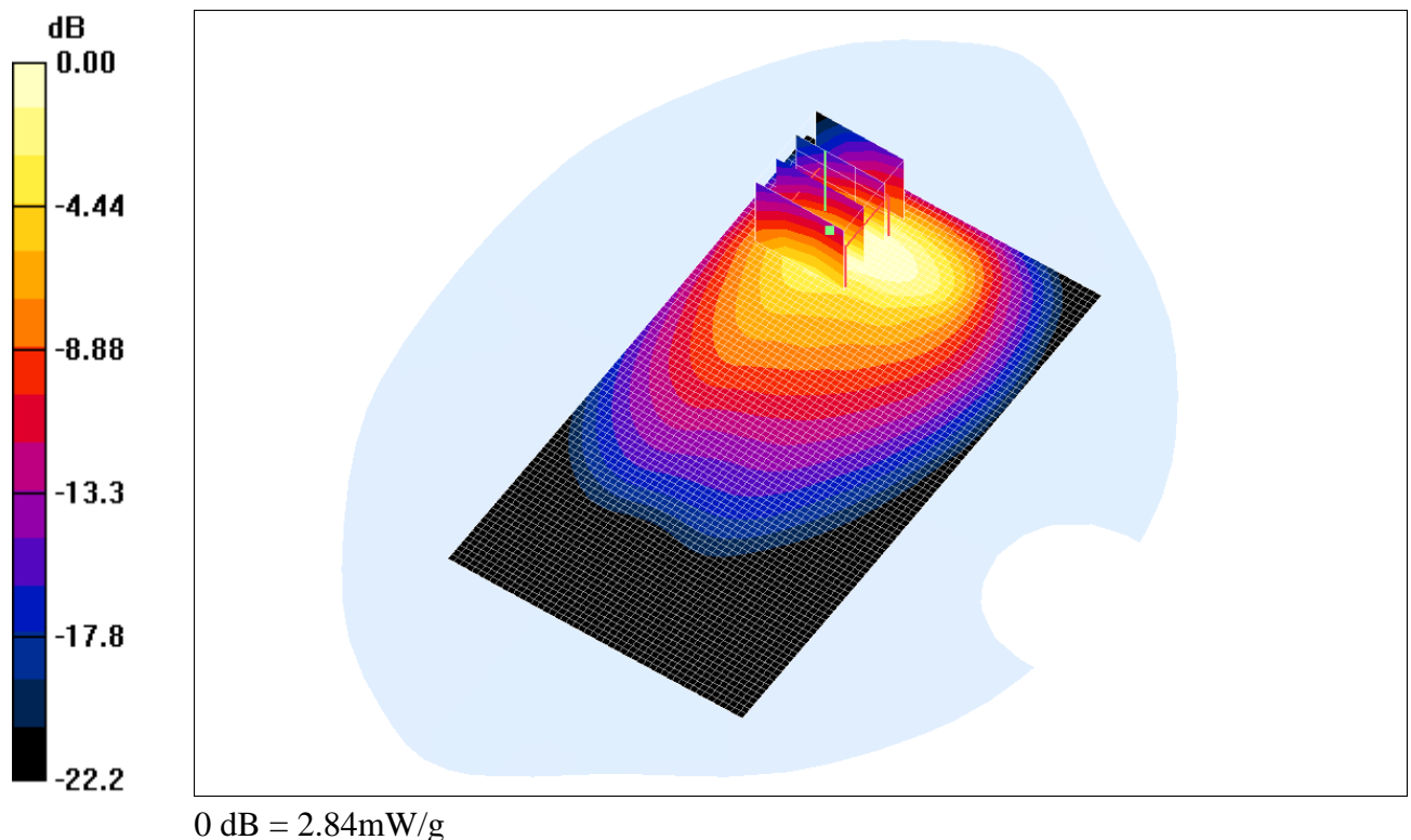
Fig. 12: Distribution du DAS en LTE 800: canal 24300 (847.0 MHz) face arrière à 0cm du fantôme
