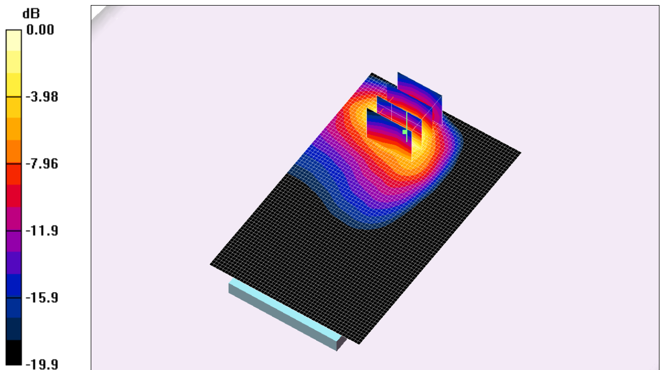
Fig. 9: Distribution du DAS en GSM-GPRS 1800: canal 512 (1710.2 MHz) face arrière à 0cm du fantôme
