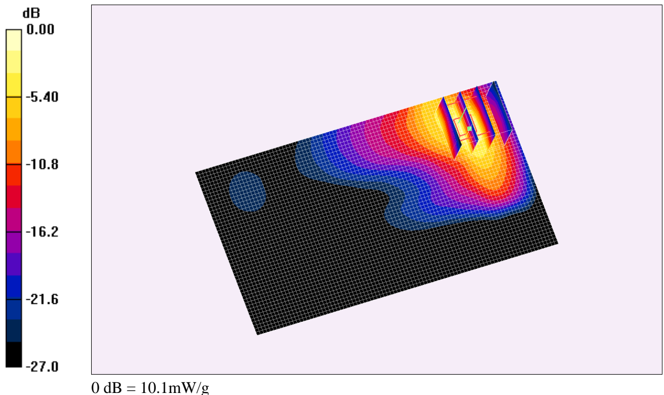
Fig. 14: Distribution du DAS en LTE 2600: canal 21350 (2560.0 MHz) face avant à 0cm du fantôme
