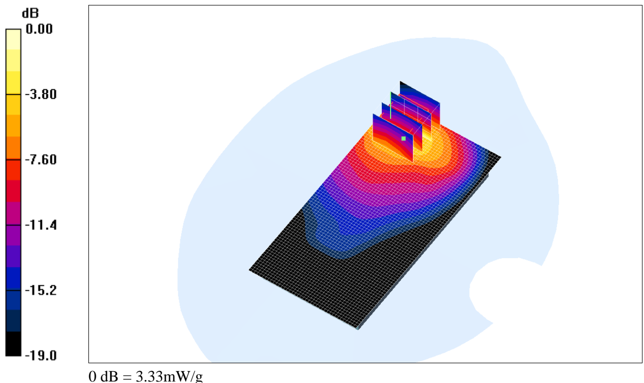
Fig. 8: Distribution du DAS en GSM-GPRS 900: canal 975 (880.2 MHz) face arrière à 0cm du fantôme
