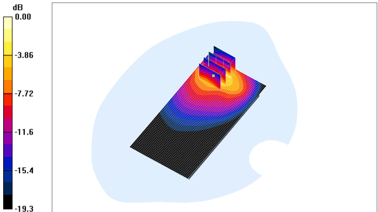
Fig. 10: Distribution du DAS en WCDMA 900: canal 2788 (897.6 MHz) face arrière à 0cm du fantôme
