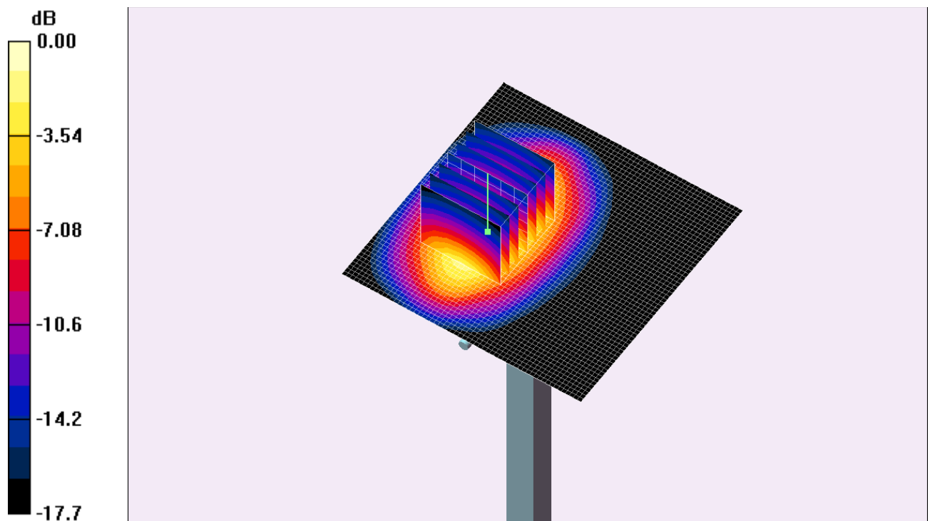
Fig. 5: Résultat de la vérification à 1800MHz
