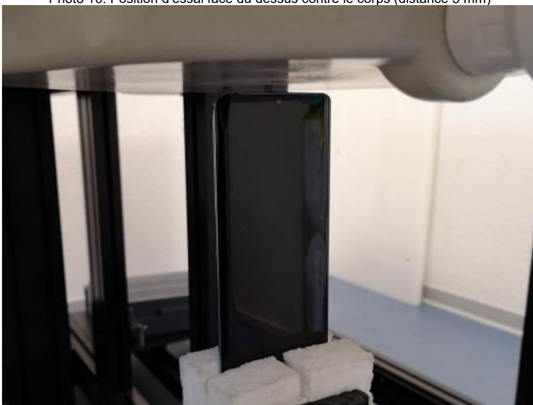
Photo 10: Position d'essai face du dessus contre le corps (distance 5 mm)
