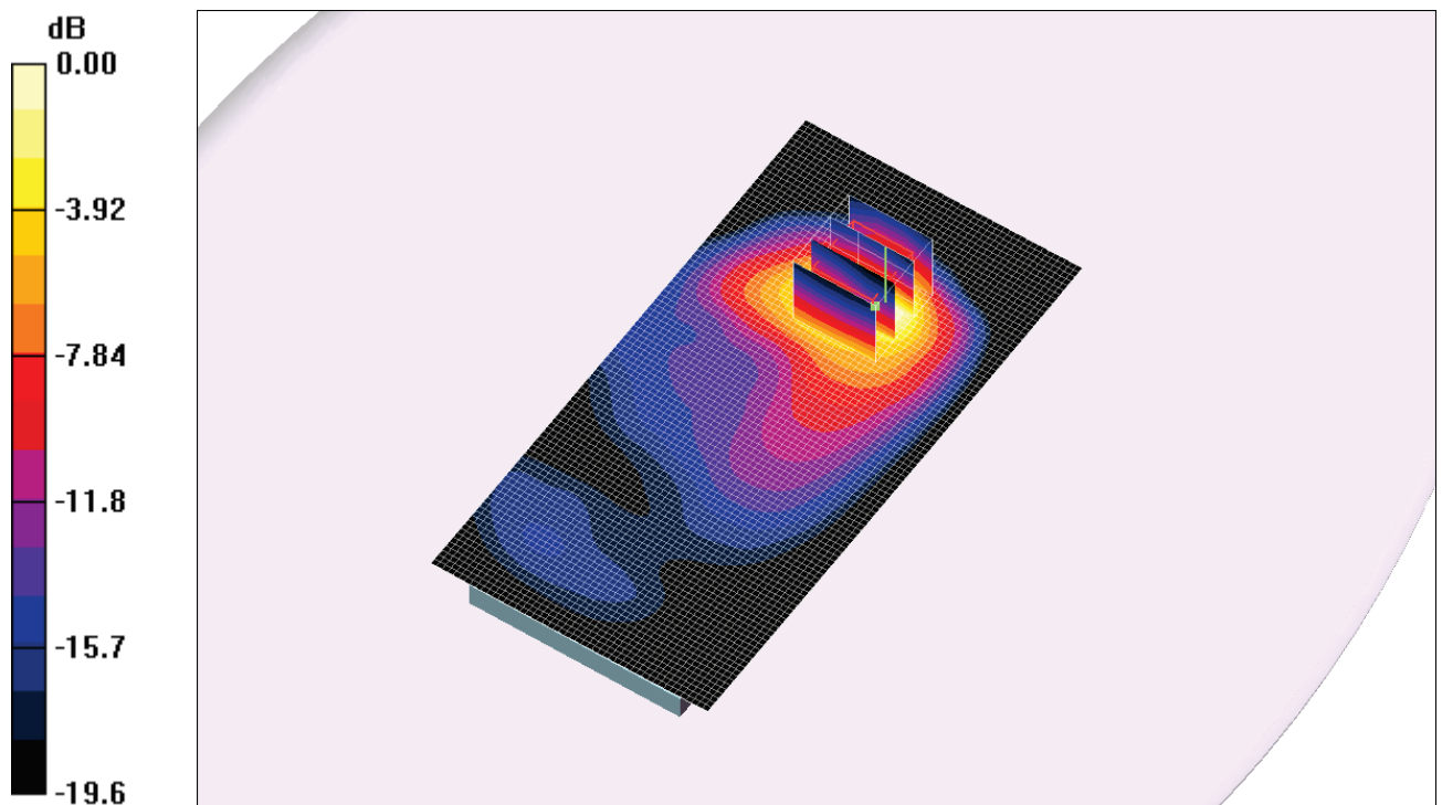
Fig. 11 : Distribution du DAS en WCDMA 2100: canal 9612 (1922.4 MHz) face avant à 0.5cm du fantôme
