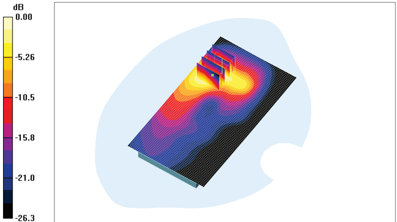
Fig. 14 : Distribution du DAS en LTE 2600: canal 21100 (2535.0 MHz) face avant à 0.5cm du fantôme
