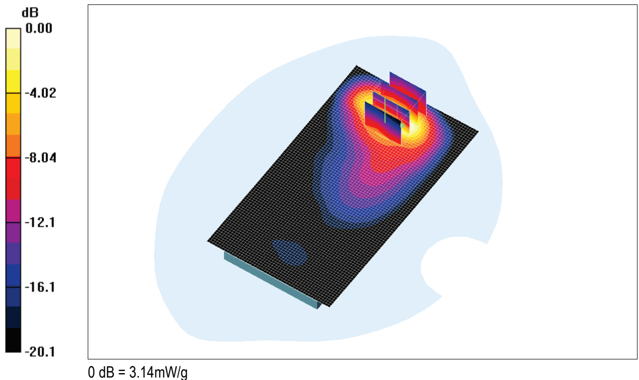
Fig. 9 : Distribution du DAS en GSM-GPRS 1800: canal 512 (1710.2 MHz) face avant à 0.5cm du fantôme
