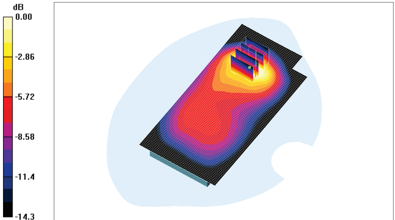
Fig. 8 : Distribution du DAS en GSM-GPRS 900: canal 038 (897.6 MHz) face avant à 0.5cm du fantôme
