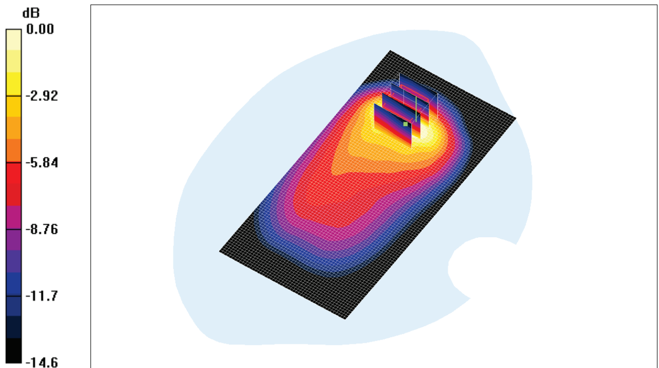
Fig. 12 : Distribution du DAS en LTE 800: canal 24250 (842.0 MHz) face avant à 0.5cm du fantôme
