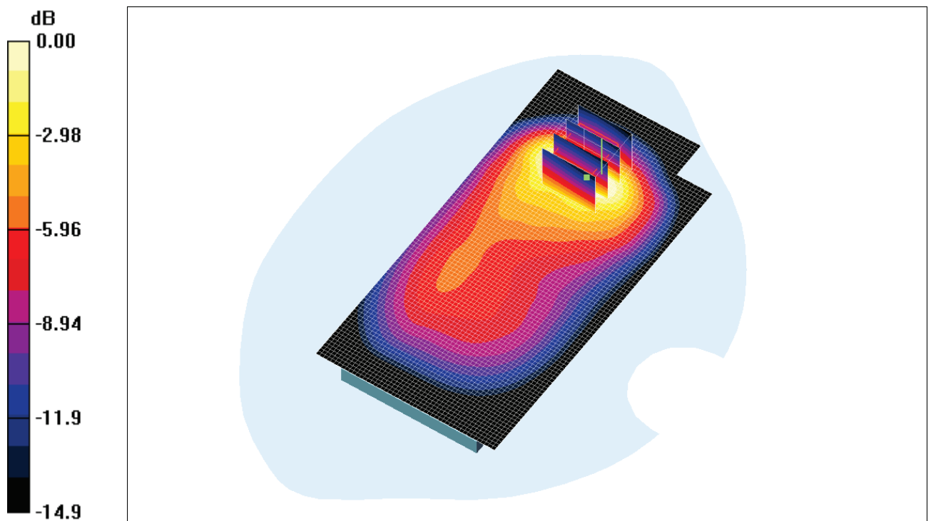
Fig. 10 : Distribution du DAS en WCDMA 900: canal 2788 (897.6 MHz) face avant à 0.5cm du fantôme
