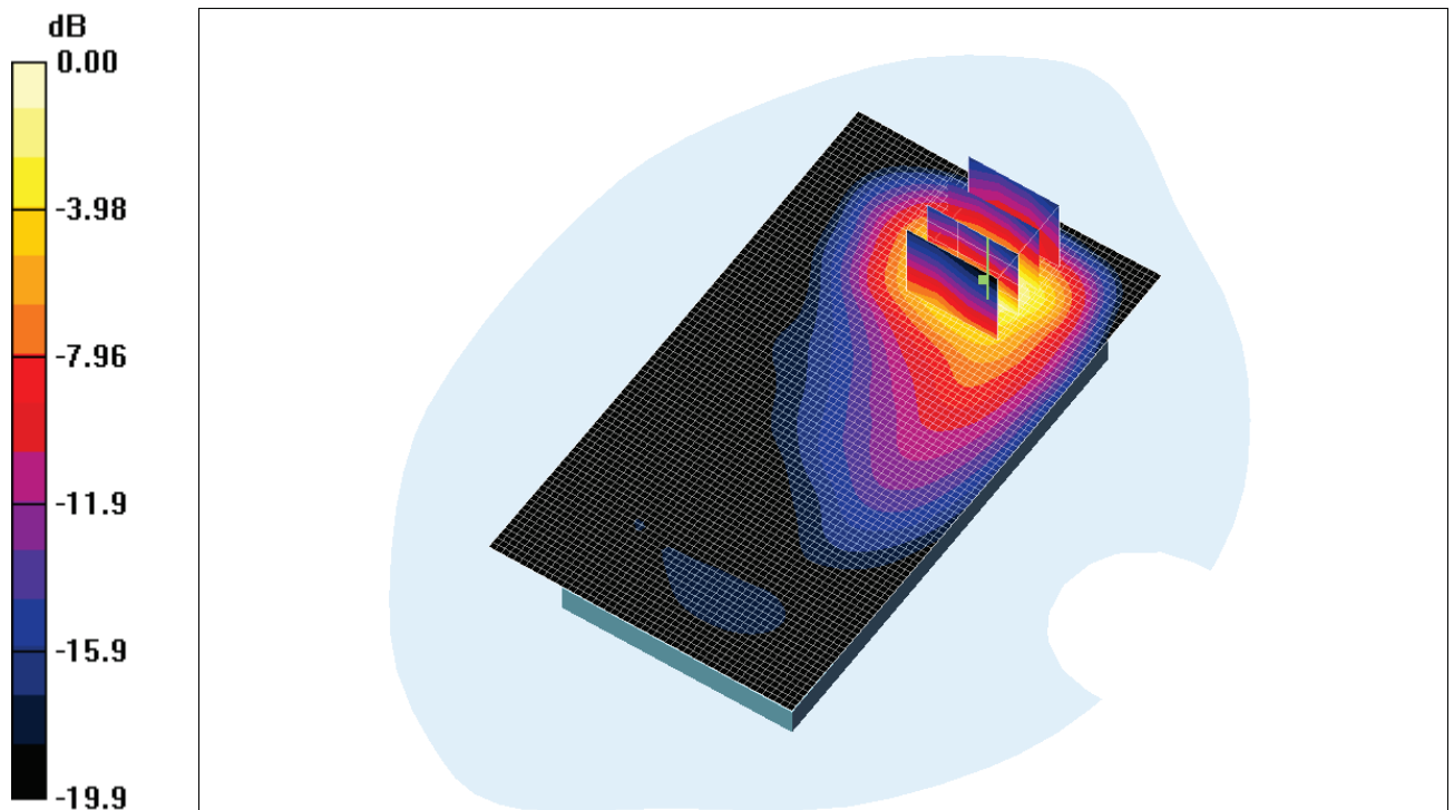
Fig. 13 : Distribution du DAS en LTE 1800: canal 19575 (1747.5 MHz) face avant à 0.5cm du fantôme
