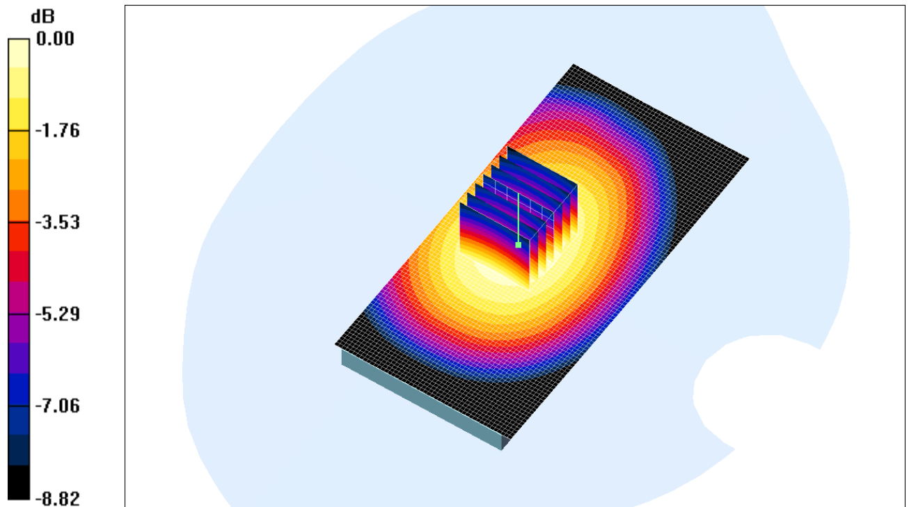
Fig. 11: Distribution du DAS en WCDMA 900: canal 2788 (897.6 MHz) face arrière à 1.5cm du fantôme
