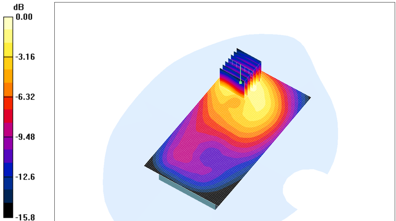
Fig. 9: Distribution du DAS en GSM-GPRS 1800: canal 699 (1747.6 MHz) face arrière à 1.5cm du fantôme
