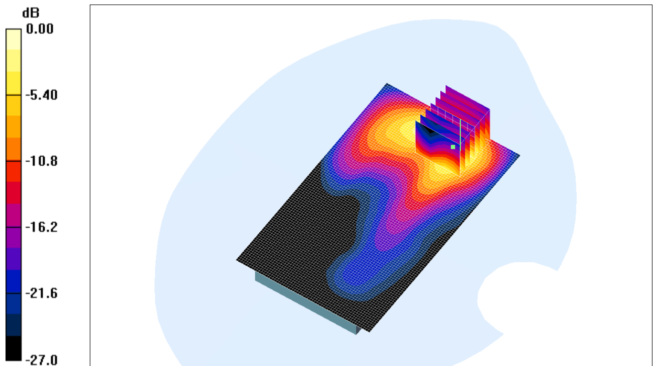
Fig. 12: Distribution du DAS en WCDMA 2100: canal 9750 (1950.0 MHz) face avant à 0cm du fantôme
