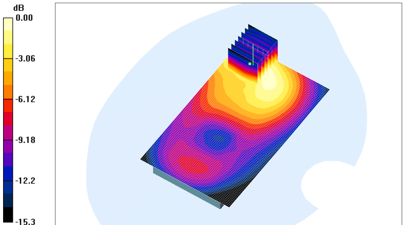
Fig. 13: Distribution du DAS en WCDMA 2100: canal 9750 (1950.0 MHz) face arrière à 1.5cm du fantôme
