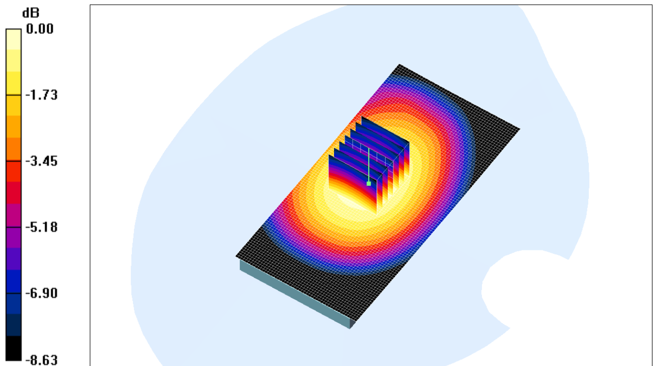
Fig. 7: Distribution du DAS en GSM-GPRS 900: canal 038 (897.6 MHz) face arrière à 1.5cm du fantôme
