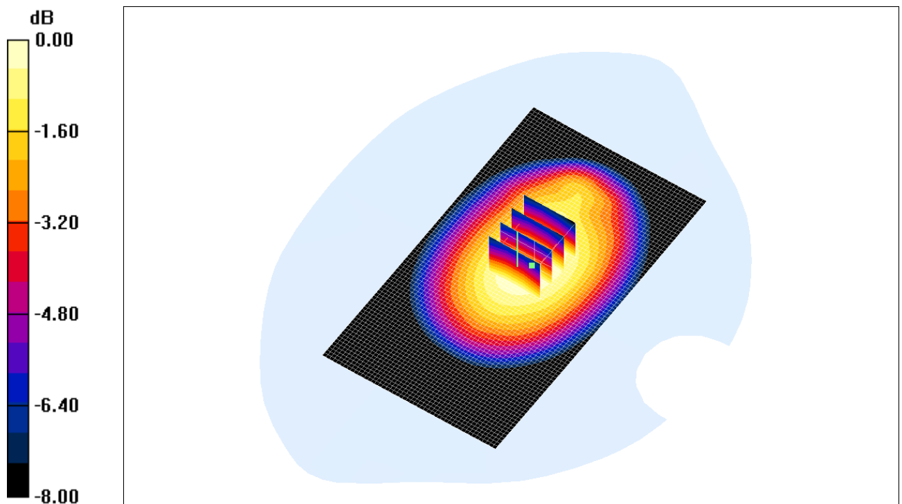
Fig. 12 : Distribution du DAS en LTE 800: canal 24175 (834.5 MHz) face arrière à 1.5cm du fantôme
