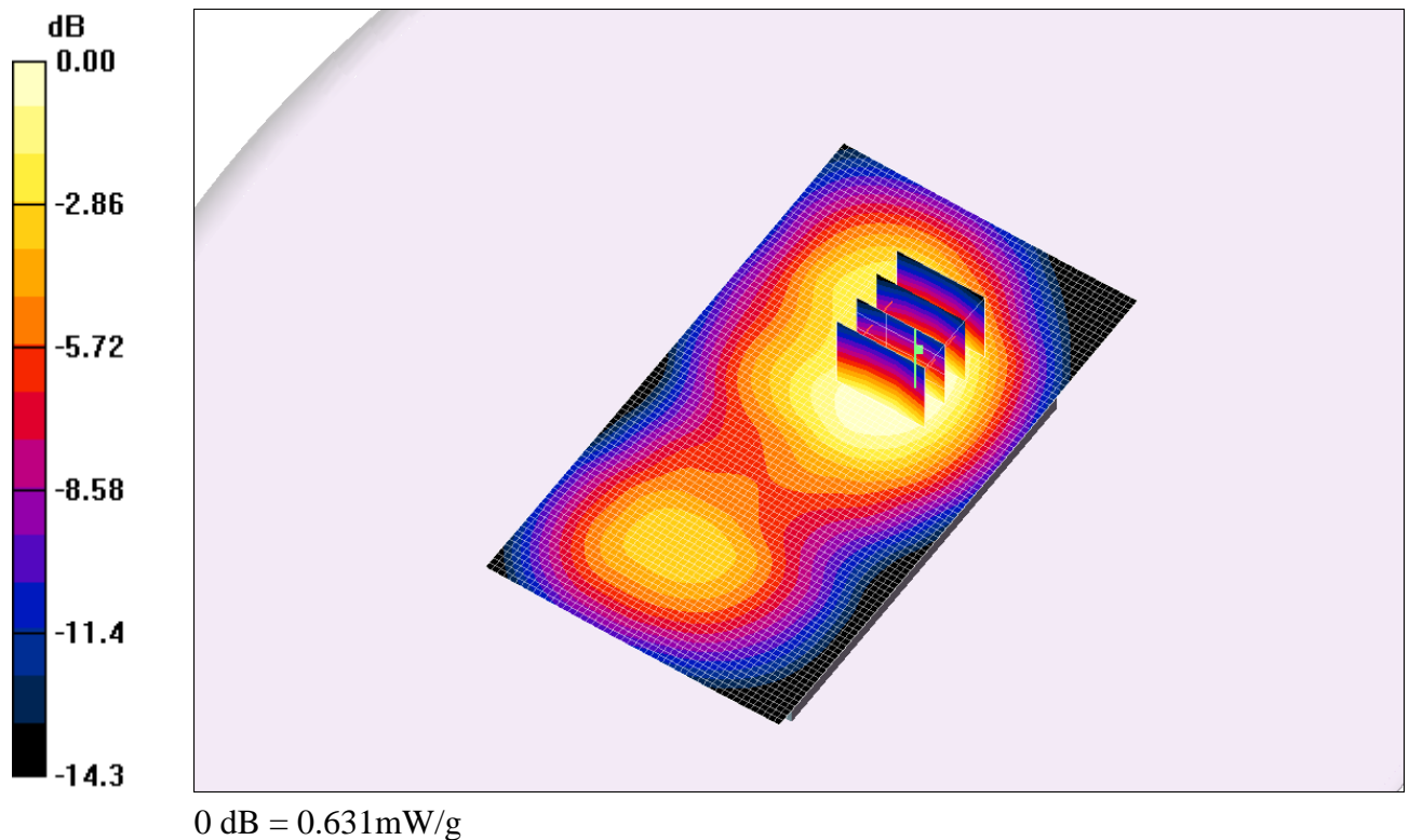
Fig. 13 : Distribution du DAS en LTE 1800: canal 19925 (1782.5 MHz) face arrière à 1.5cm du fantôme
