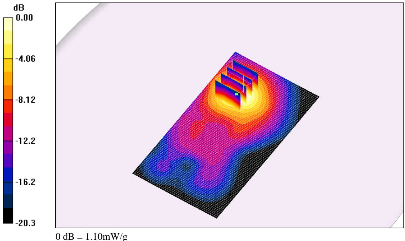
Fig. 14 : Distribution du DAS en LTE 2600: canal 21100 (2535.0 MHz) face arrière à 1.5cm du fantôme
