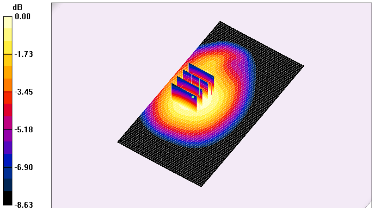
Fig. 10 : Distribution du DAS en WCDMA 900: canal 2863 (912.6 MHz) face arrière à 1.5cm du fantôme
