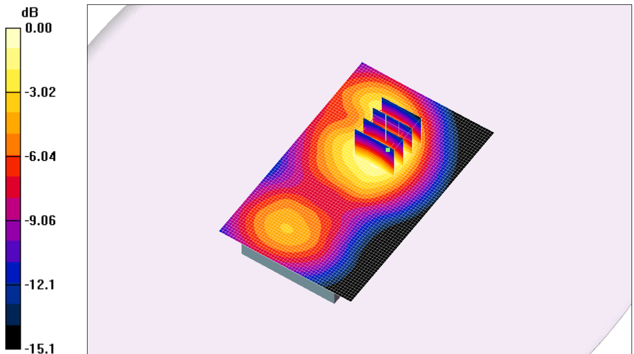
Fig. 9 : Distribution du DAS en GSM-GPRS 1800: canal 885 (1784.8 MHz) face arrière à 1.5cm du fantôme
