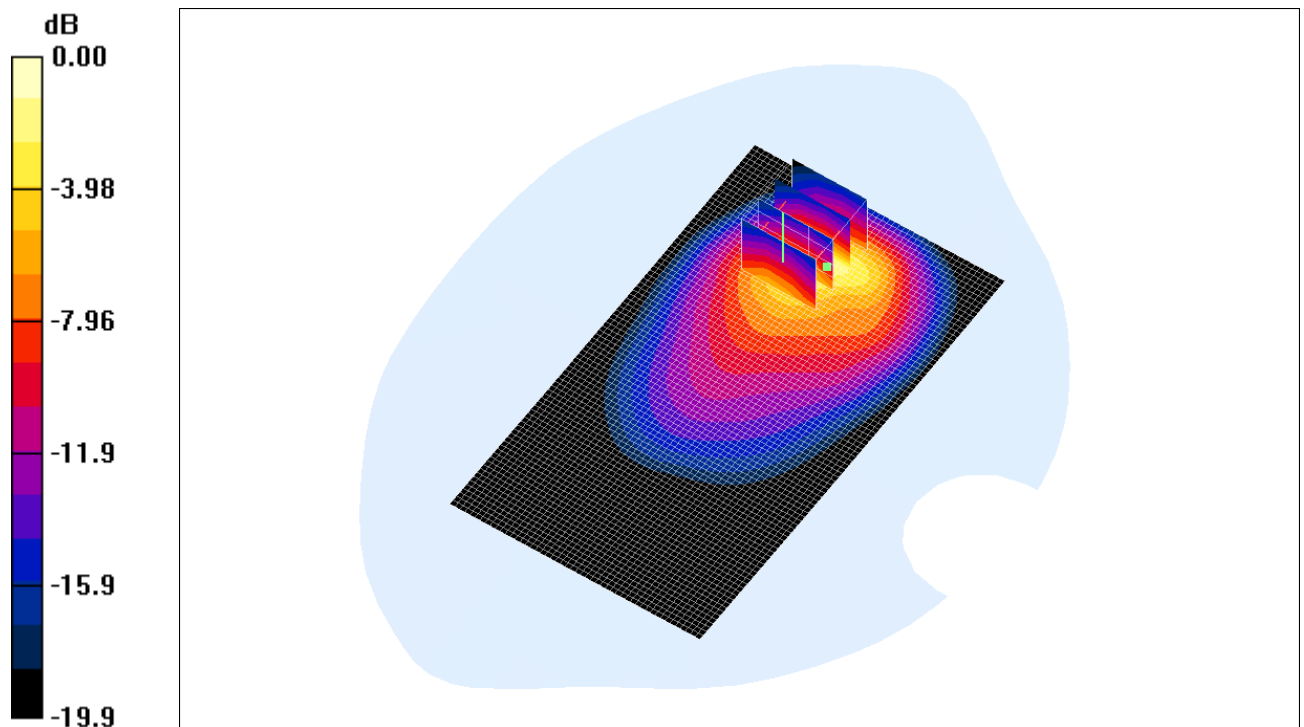
Fig. 8: Distribution du DAS en GSM-GPRS 900: canal 124 (914.8 MHz) face arrière à 0cm du fantôme
