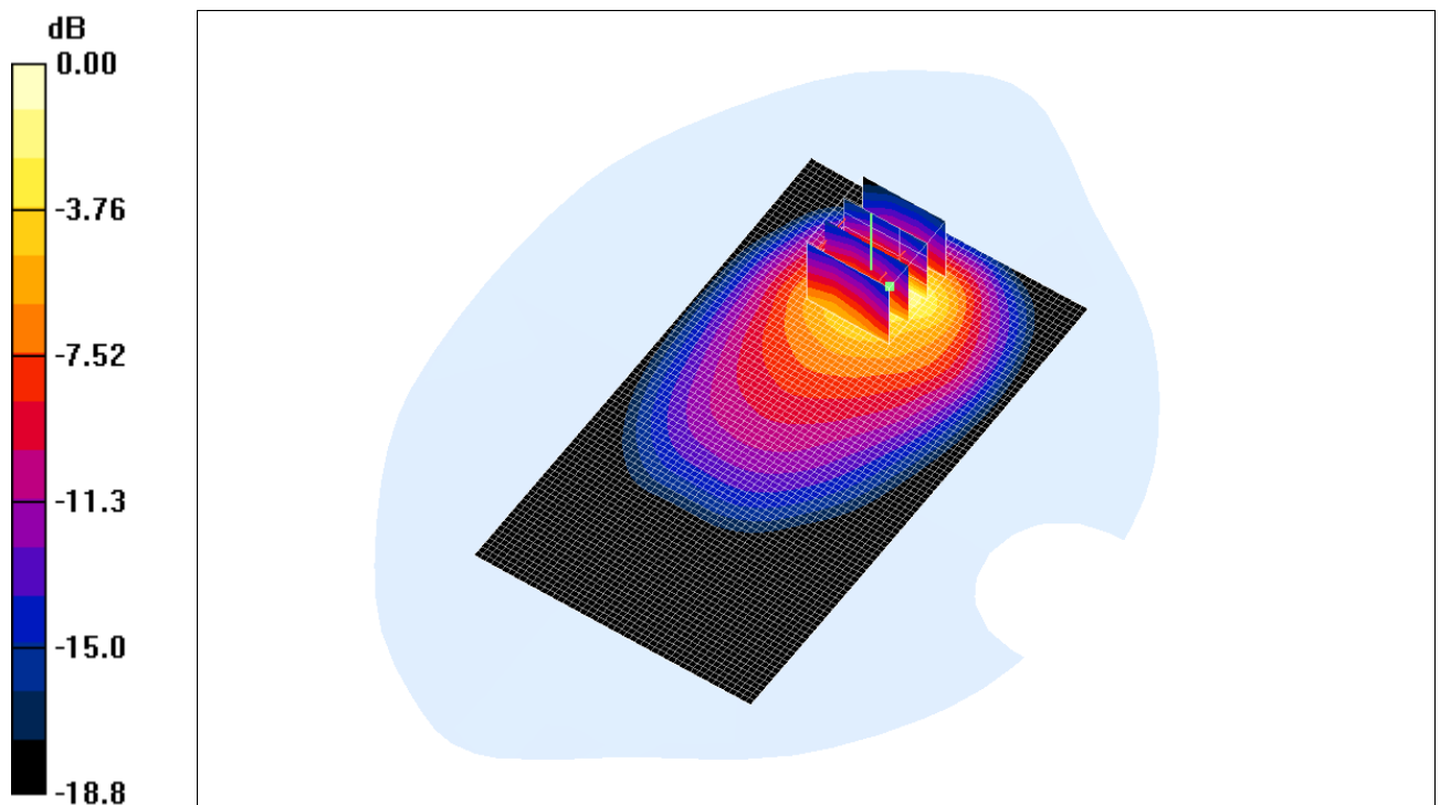
Fig. 12: Distribution du DAS en LTE 800: canal 24175 (834.5 MHz) face arrière à 0cm du fantôme
