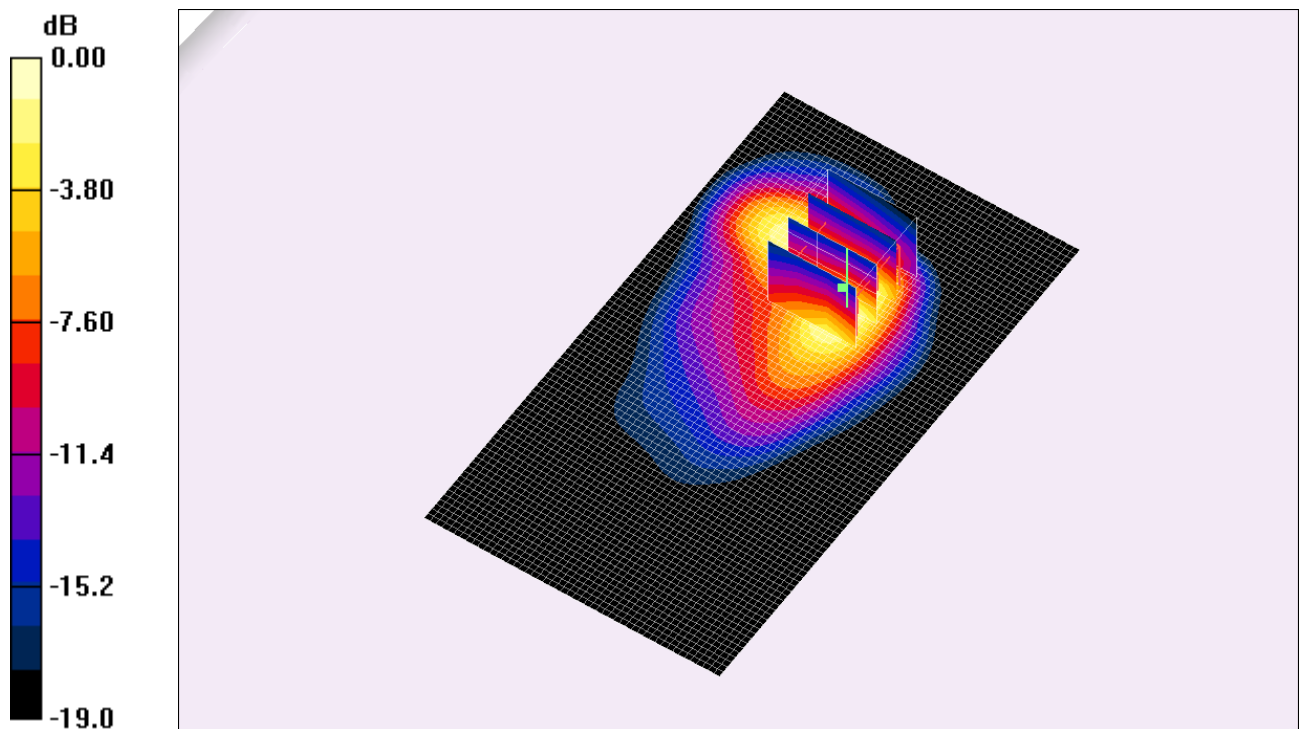
Fig. 11: Distribution du DAS en WCDMA 2100: canal 9612 (1922.4 MHz) face arrière à 0cm du fantôme
