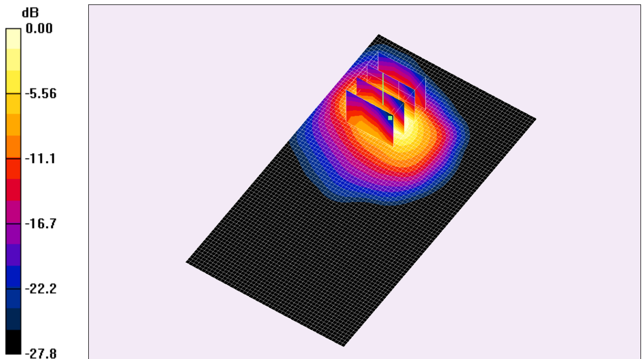
Fig. 14: Distribution du DAS en LTE 2600: canal 21100 (2535.0 MHz) face arrière à 0cm du fantôme
