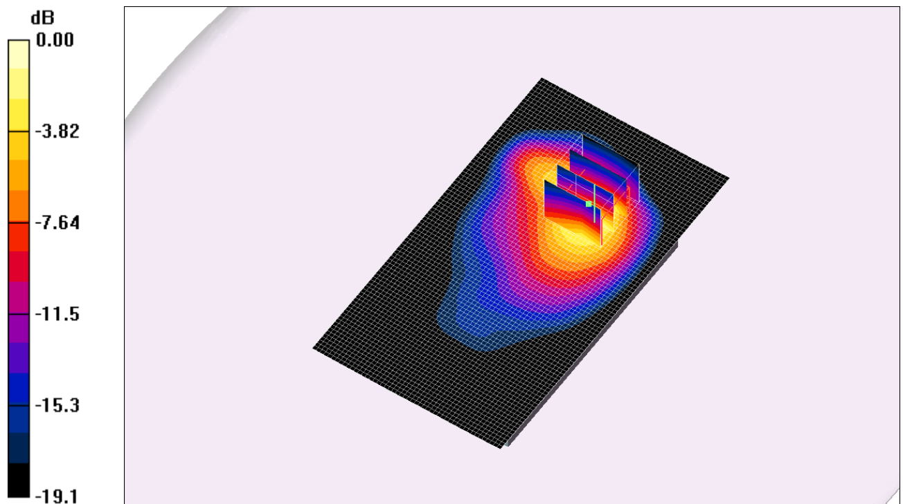
Fig. 13: Distribution du DAS en LTE 1800: canal 19925 (1782.5 MHz) face arrière à 0cm du fantôme
