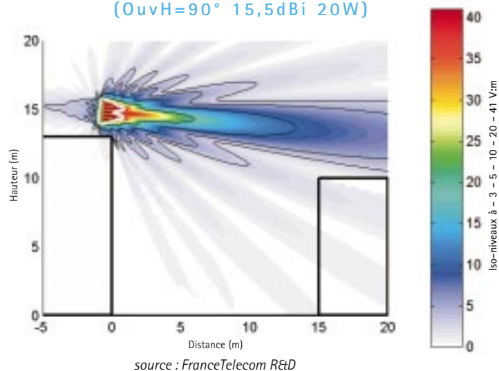
Site Macro sur Terrasse - Vue Verticale (OuvH=90° 15,5dBi 20W)
